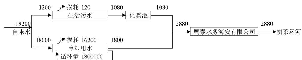
图 2-1 本项目营运期水平衡图（单位：t/a）
