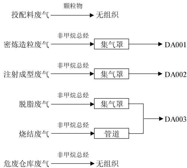
图 4-1 本项目废气收集、处理方式示意图
