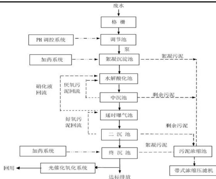
图 4-2 鹰泰水务海安有限公司工艺流程图
