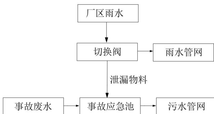
图 4-7 事故废水收集系统图
